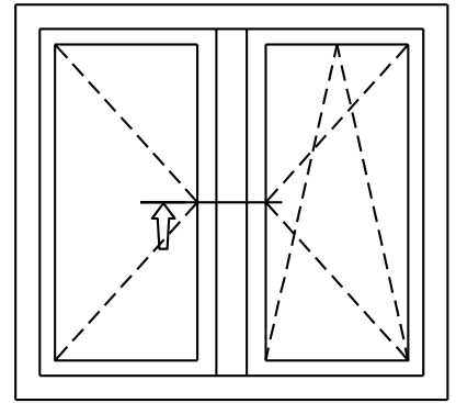
IV62 WOOD/WOOD SEZIONE ORIZZONTALE CHIUSURA CENTRALE HORIZONTAL SECTION OF THE MIDDLE CLAMP
